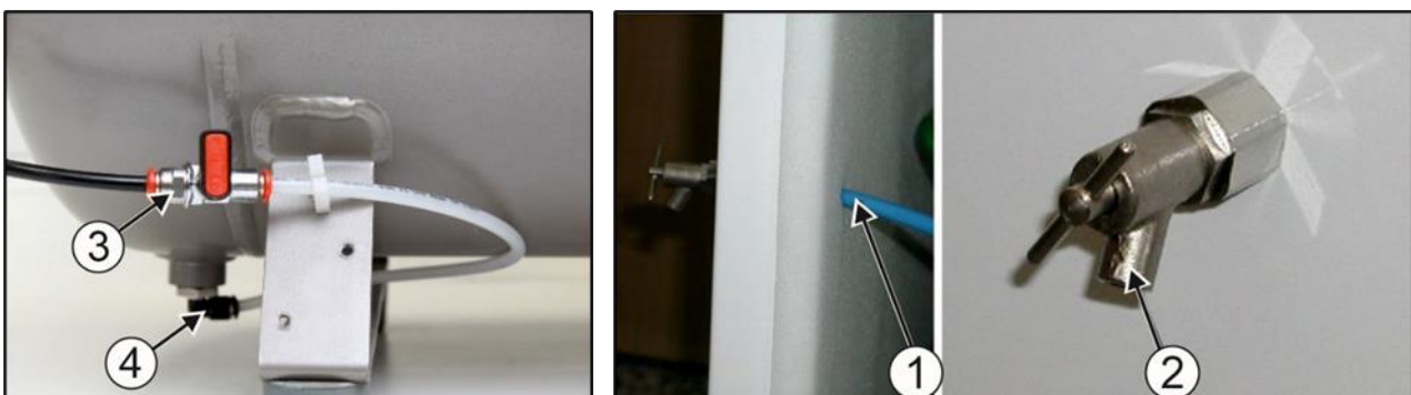
Obr. 7: Osadenie ventilu na odvod kondenzátu na skrinku
